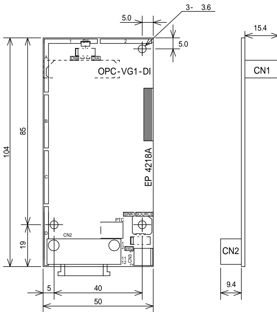
図 1.2-1 インタフェースカード外形
